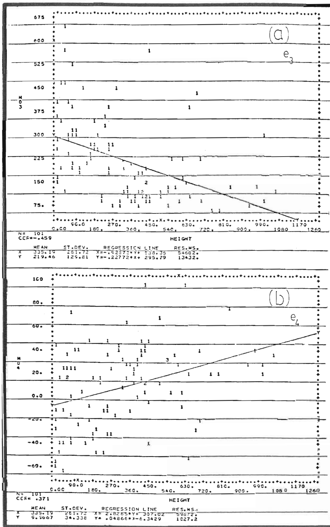
Figura 13.—Gráfico de regresión lineal entre la elevación (m) y el coeficiente del eigenvector cronológico (a): e_3 y (b): e_4 para cada puesto.
