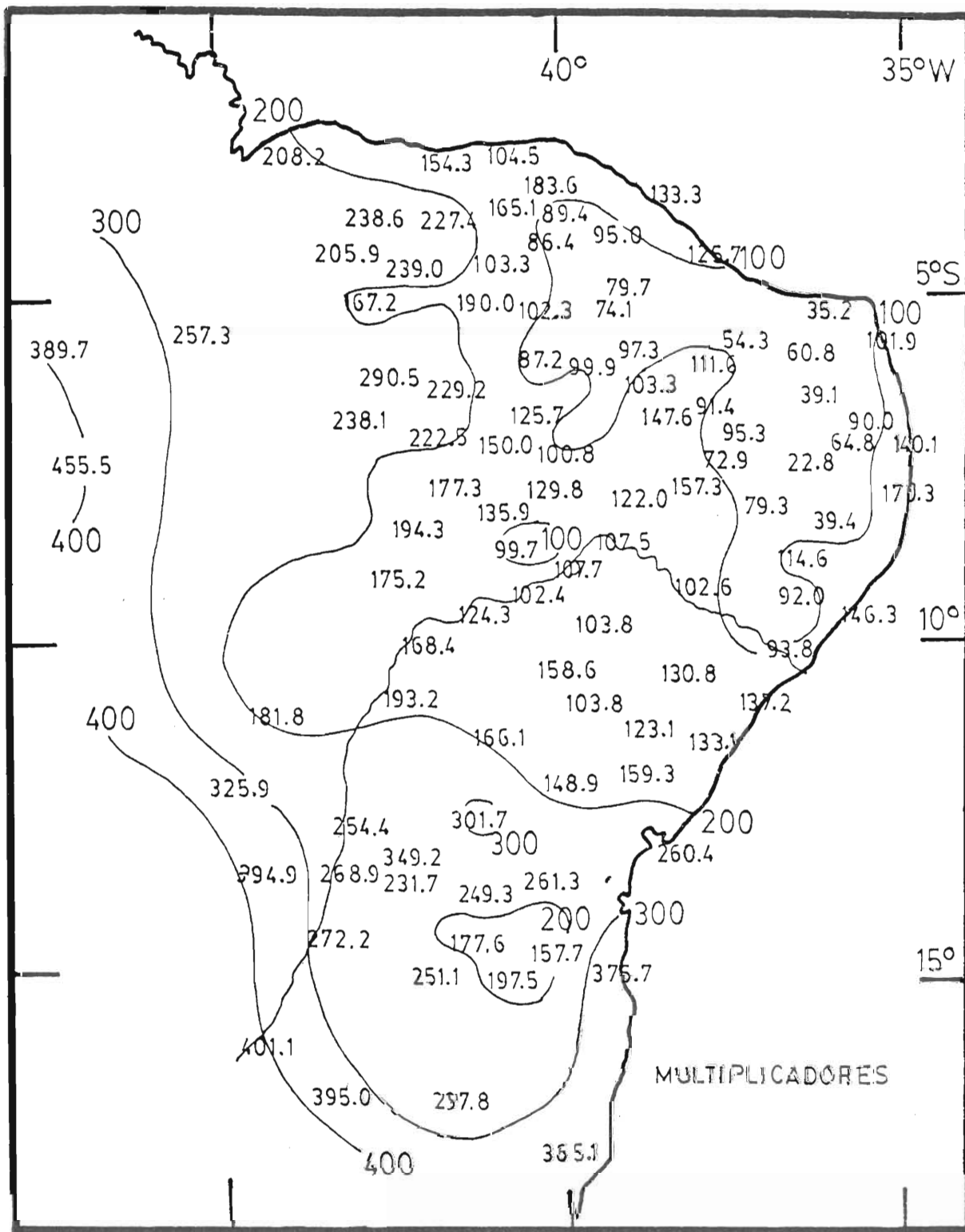
Figura 9.—Distribución geográfica de los multiplicadores del segundo vector propio cronológico.
