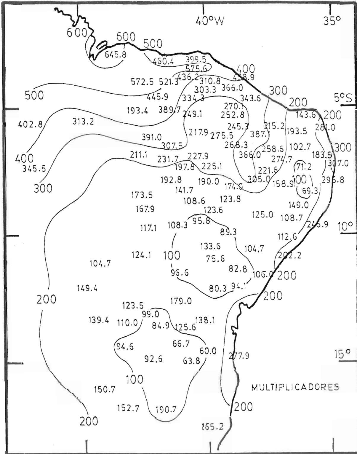
Figura 10.—Distribución geográfica de los multiplicadores del tercer vector propio cronológico.
