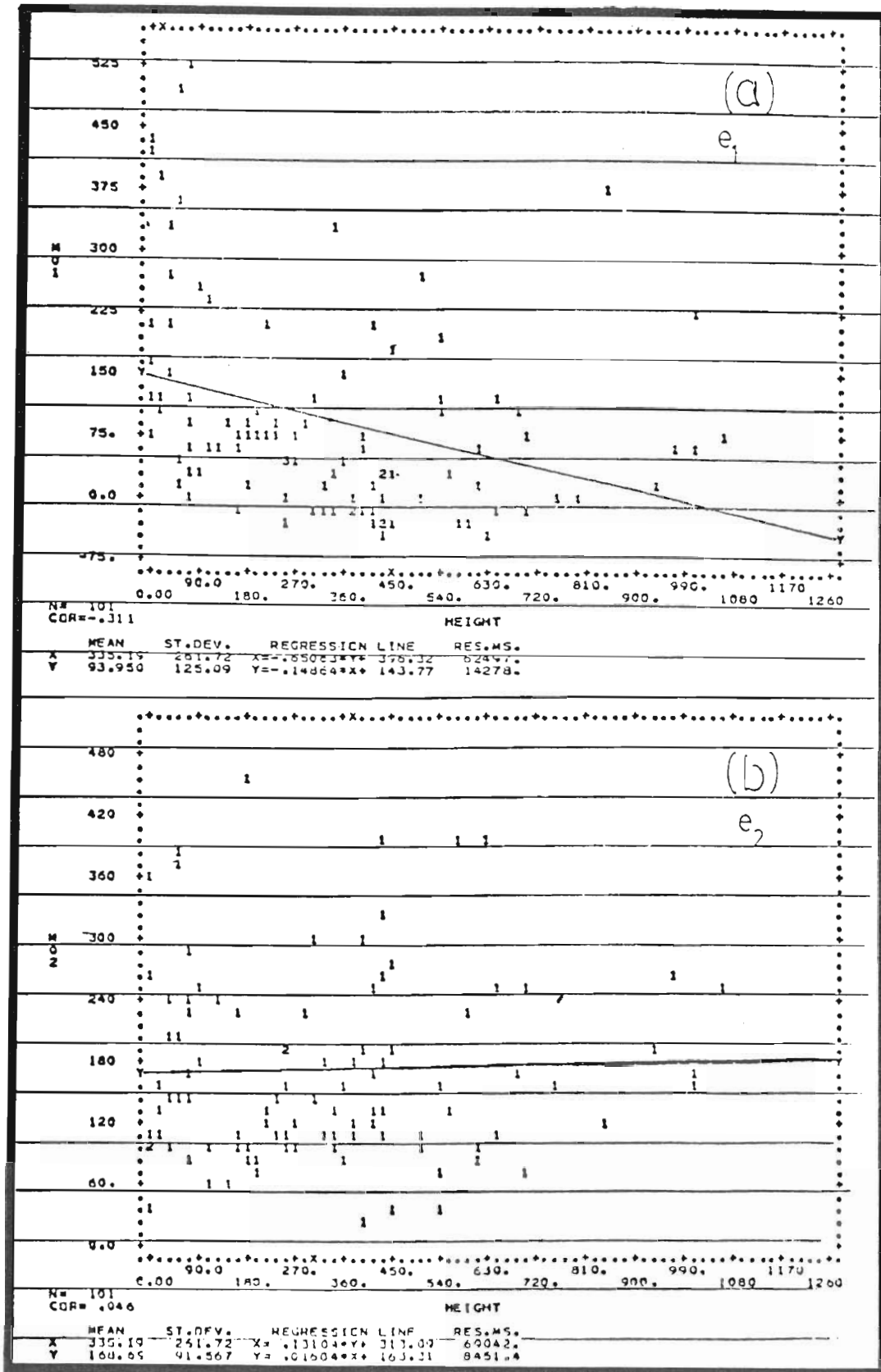
Figura 12.—Gráfico de regresión lineal entre la elevación (m) y el coeficiente de eigenvector cronológico (a): e_1 y (b): e_2 para cada puesto.
