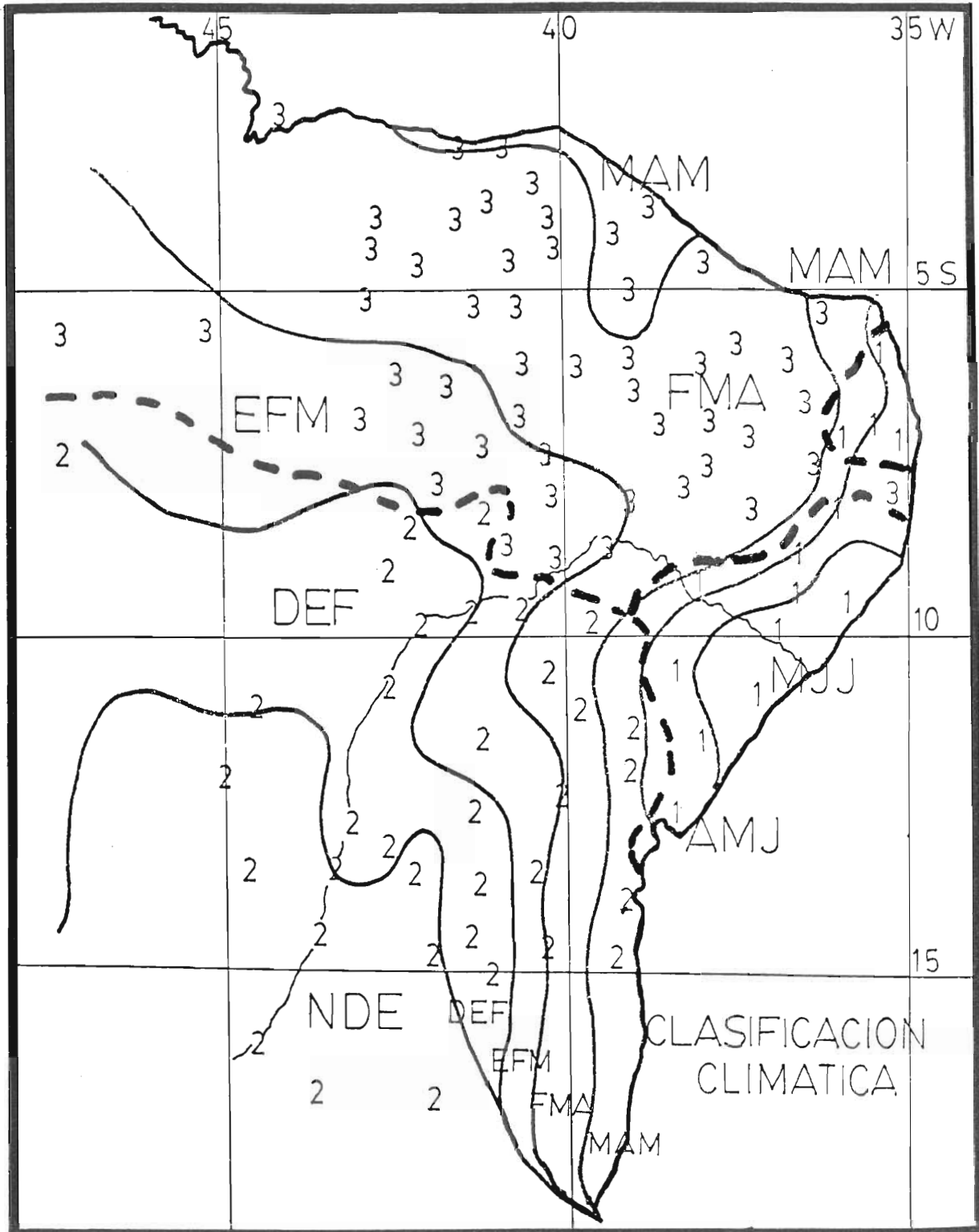
Figura 6.—Clasificación pluvioclimática objetiva para el nordeste (ver texto). Línea de trazos: límites de las regiones. Líneas continuas: límites de los totales trimestrales máximos y meses de ocurrencia (iniciales).
