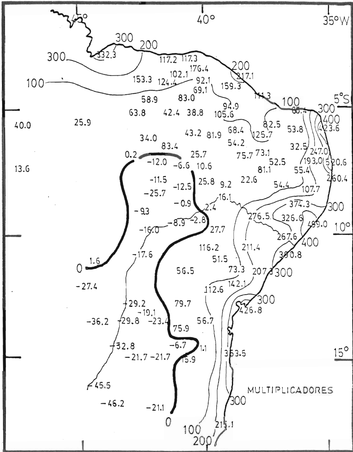
Figura 8.—Distribución geográfica de los multiplicadores del primer vector propio cronológico.
