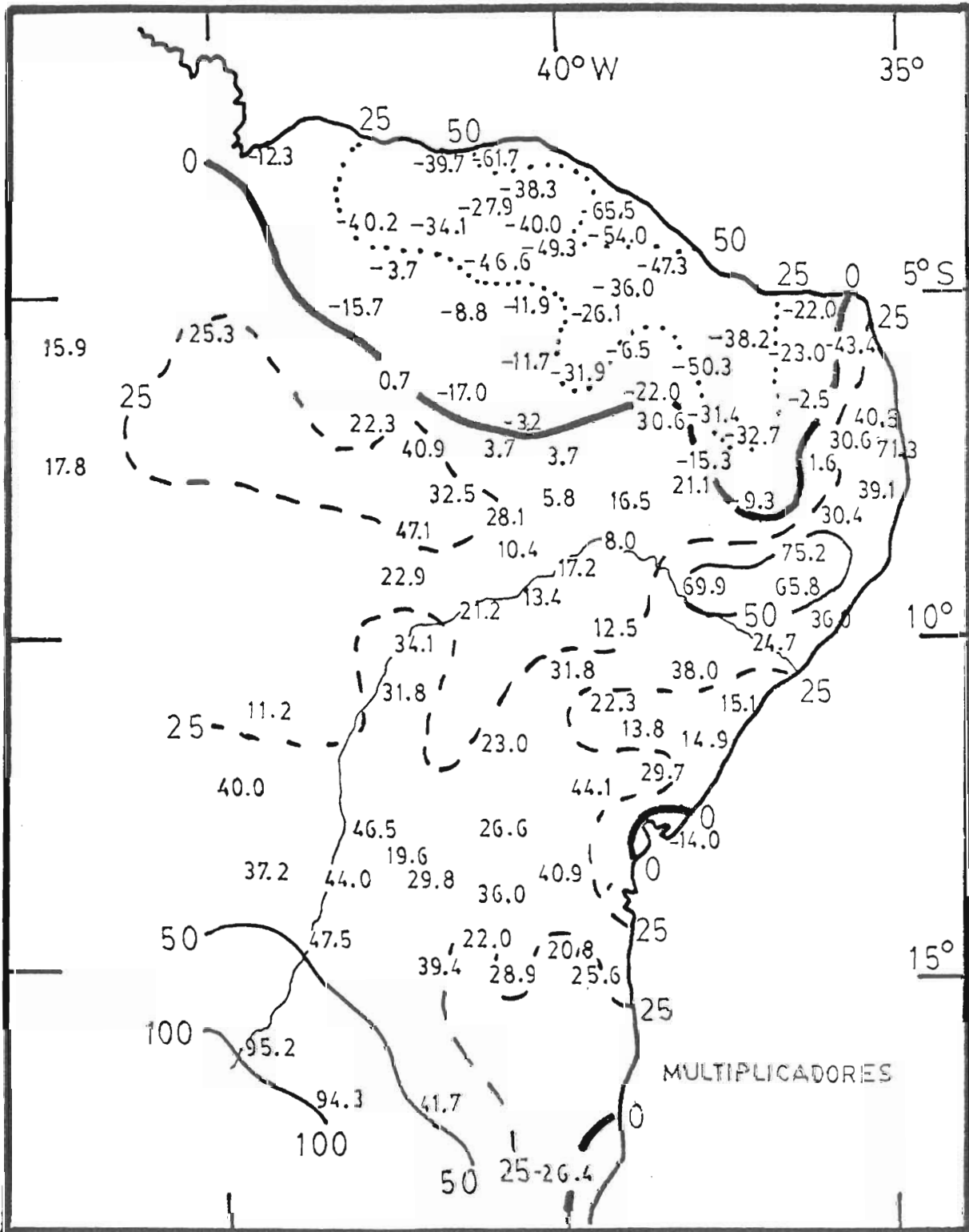
Figura 11.—Distribución geográfica de los multiplicadores del cuarto vector propio cronológico.
