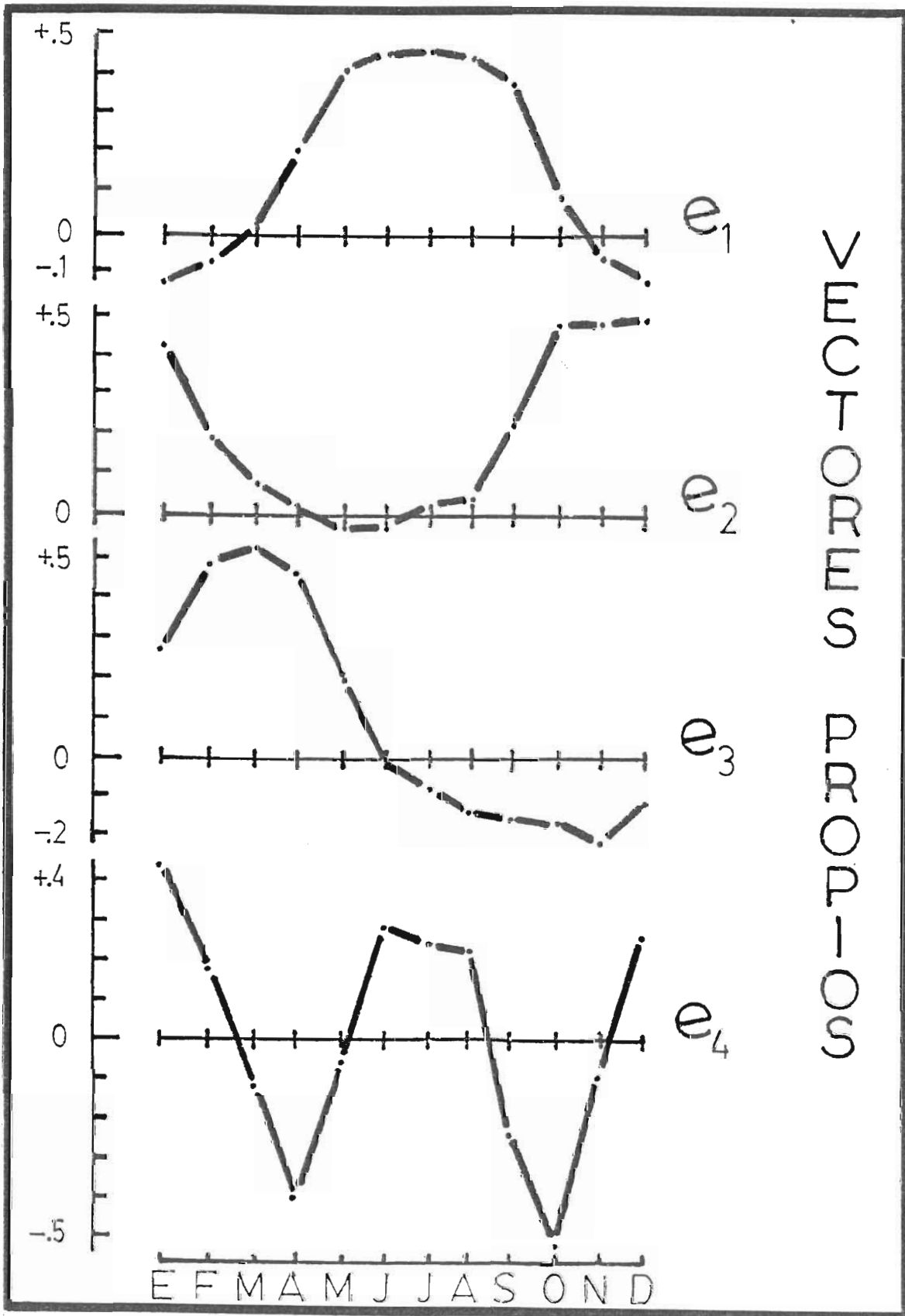
Figura 5.—Los cuatro primeros vectores propios cronológicos.
