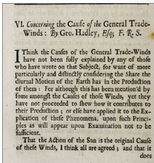
Inicio del artículo “Concerning the Cause of the Trade Winds” de George Hadley, publicado en 1735 (fuente: http://rstl.royalsocietypublishing.org/content/39/437/58 )
