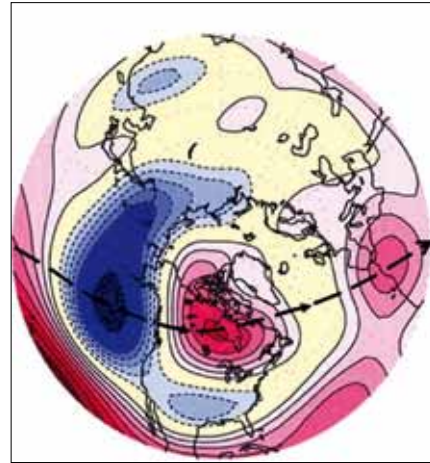
Figura 3. Proyección polar de las anomalías del geopotencial en 200 hPa para dic-ene-feb en el hemisferio norte en situaciones de El Niño. Altas en rojo (anticiclónicas) y bajas en azul (cyclónicas).
