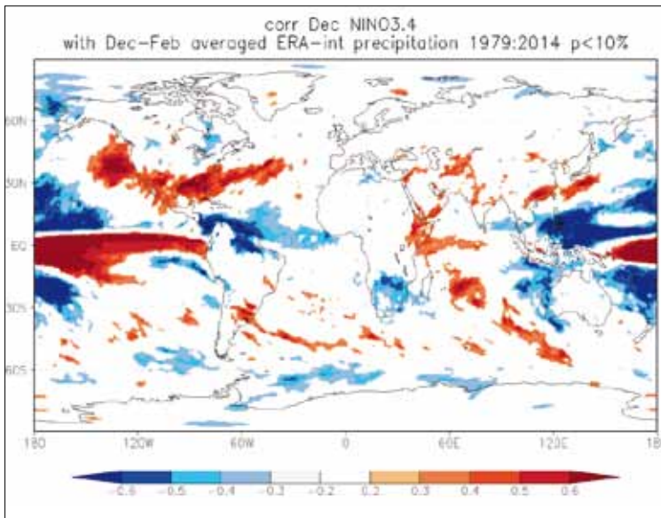
Figura 4. Correlación precipitación-índice Niño3.4 para el periodo DEF, usando datos de ERA Interim. Mapa obtenido en https://climexp.knmi.nl/
