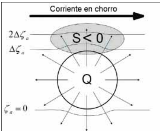
Figura 2. Esquema de zona de generación de ondas de Rossby en las capas altas de la troposfera ( |S| > 0 ) por la interacción del flujo divergente sobre la convección tropical (flechas), con el gradiente de la vorticidad absoluta (contornos finos) en las proximidades del chorro subtropical.
