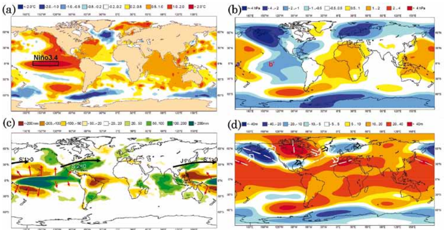
Figura 1. Mapas de anomalías medias previstos (+1mes) para dic-ene-feb de: (a) temperatura de la superficie del mar (marcada región NIÑO3.4); (b) presión al nivel del mar (a' - b' dipolo de presión en el Pacífico ecuatorial); (c) precipitación (S'1 y S'2 regiones de anomalías de fuentes de Rossby del Pacífico norte y del Golfo de México; flechas en rojo y negro: esquemas de viento divergente y corrientes en chorro subtropicales en niveles altos); (d) geopotencial en 500 hPa (esquematisados trenes de ondas de Rossby; en blanco el asociado a S'1; en negro el asociado a S'2)
