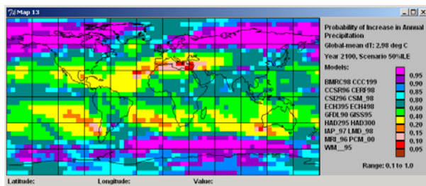
Fig.11.- Probabilidad de aumento de precipitación anual media obtenida mediante MAGICC-SCENGEN (versión 4.1) promediando 17 AOGCMs y para el percentil 50% de los escenarios de emisión SRES-IPCC.
