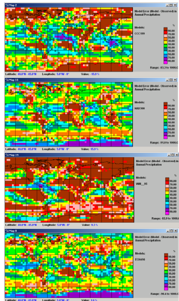
Fig.7.- Error medio de la precipitación anual en el periodo de referencia para los modelos CCC199, HAD300, WM_95 y ECH498 (producido con MAGICC-SCENGEN, version 4.1).
