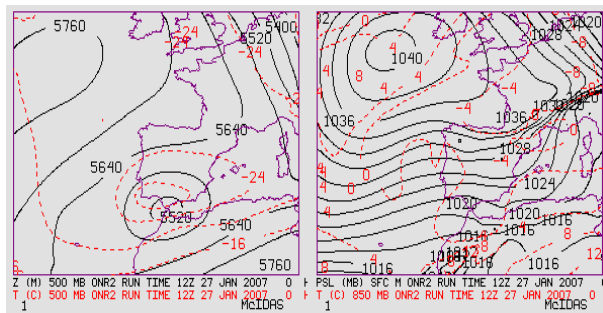
Fig. 6.- Análisis Hirlam básico de Z, T 500 hPa, y PSL y T 850 hPa. 27 Enero a 12 Z.
