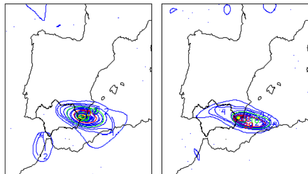
Fig. 7.- Precipitación prevista desde el día anterior por el modelo del ECWMF de 6 en 6 horas para el día 27
