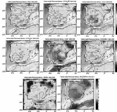
Fig. 2.- Campos de velocidades medias anuales del viento sobre la Península Ibérica para el periodo de tiempo 1989-2008. Para los modelos del proyecto ESCENA y las bases de referencia de datos climáticos de reanálisis ERA-Interim y MERRA.
