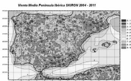
Fig. 1.- Campos de velocidades medias anuales del viento sobre la Península Ibérica para el periodo de tiempo 2004-2011, para el modelo SKIRON.
